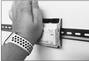
Gerät auf Hutschiene drücken
